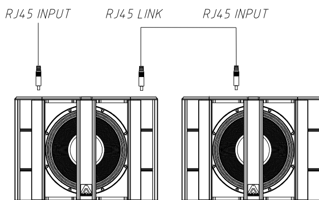
Fig.12. Conexión en paralelo para XW118 (Ethernet). Máximo ocho unidades linkadas.
